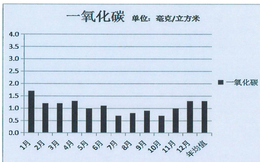
一氧化碳月平均浓度变化图
